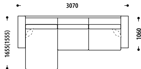
PLM,OTL-2M L+600mm,PPM
