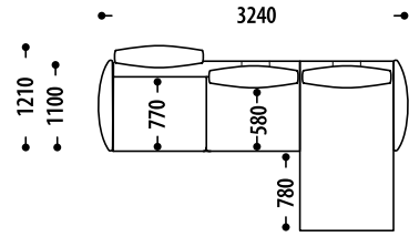
2MrL-OTPL L-150mm
